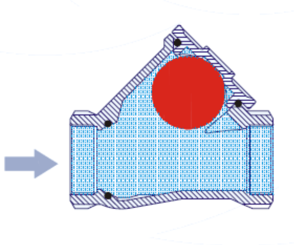
Montage Horizontal
