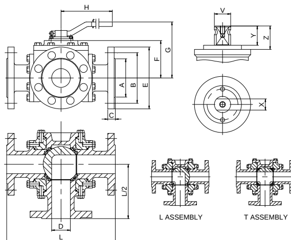
FIG.Z 86 TTT PN40 DN25-100 L/T
