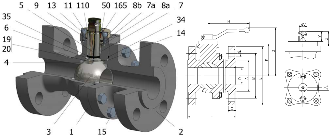
FIG.Z 64 SSSGV CL600 1/2"-2"
