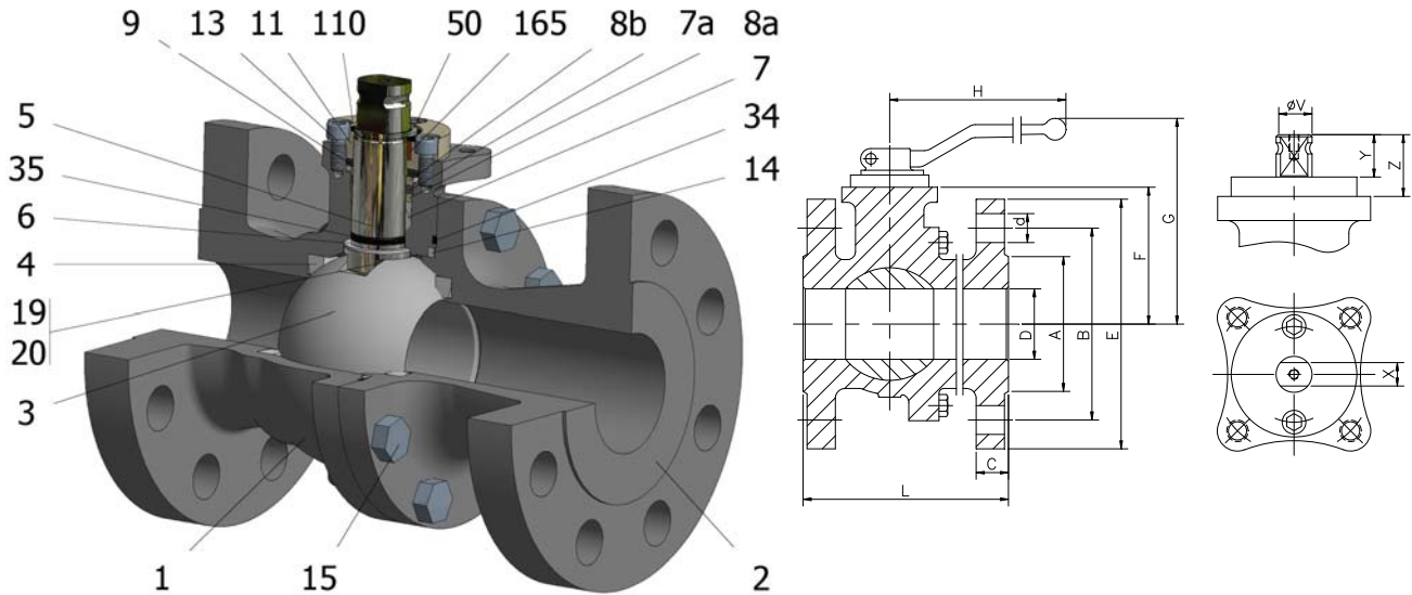
FIG.Z 34 SSSGV CL300 1/2"-4"
