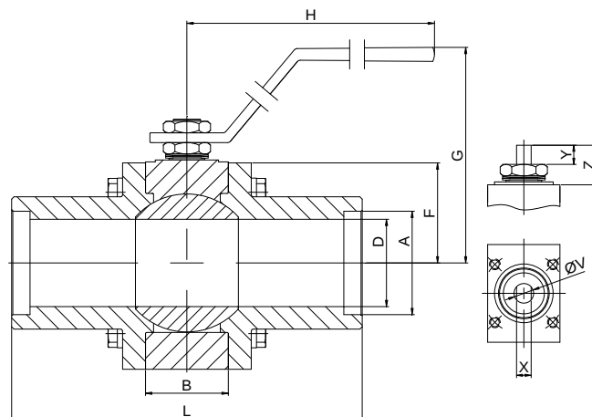
FIG.K 809 SGSGV CL400 3" SW
