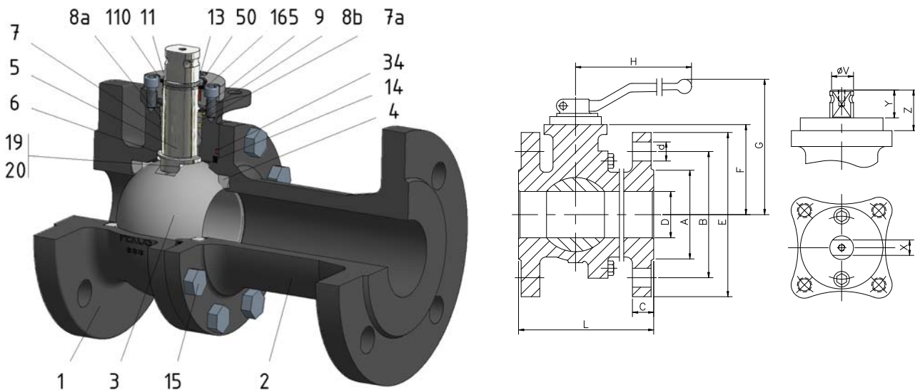
FIG.Z 29 TTTG PN16 DN15/200 F1
