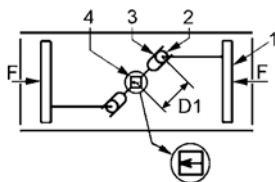
Fig. 1 - Représenté fermé
