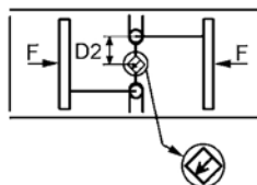
Fig. 2 - Représenté à 45°
