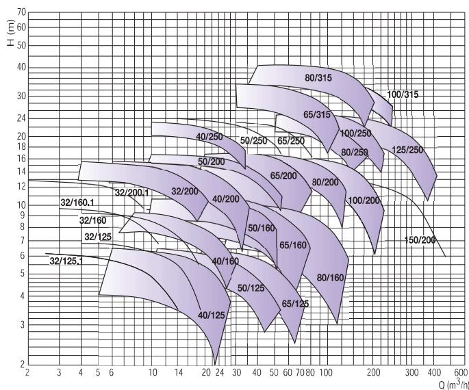
NKM 1 450 tr/min
