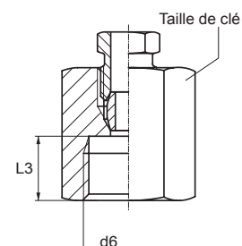
Raccord coulissant à vis femelle
