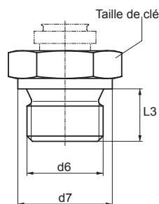
Filetages cylindriques
