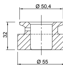
Pièce à souder sur réservoir code : 11043353
