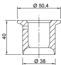
Pièce à souder sur tuyauterie code : 11039934
